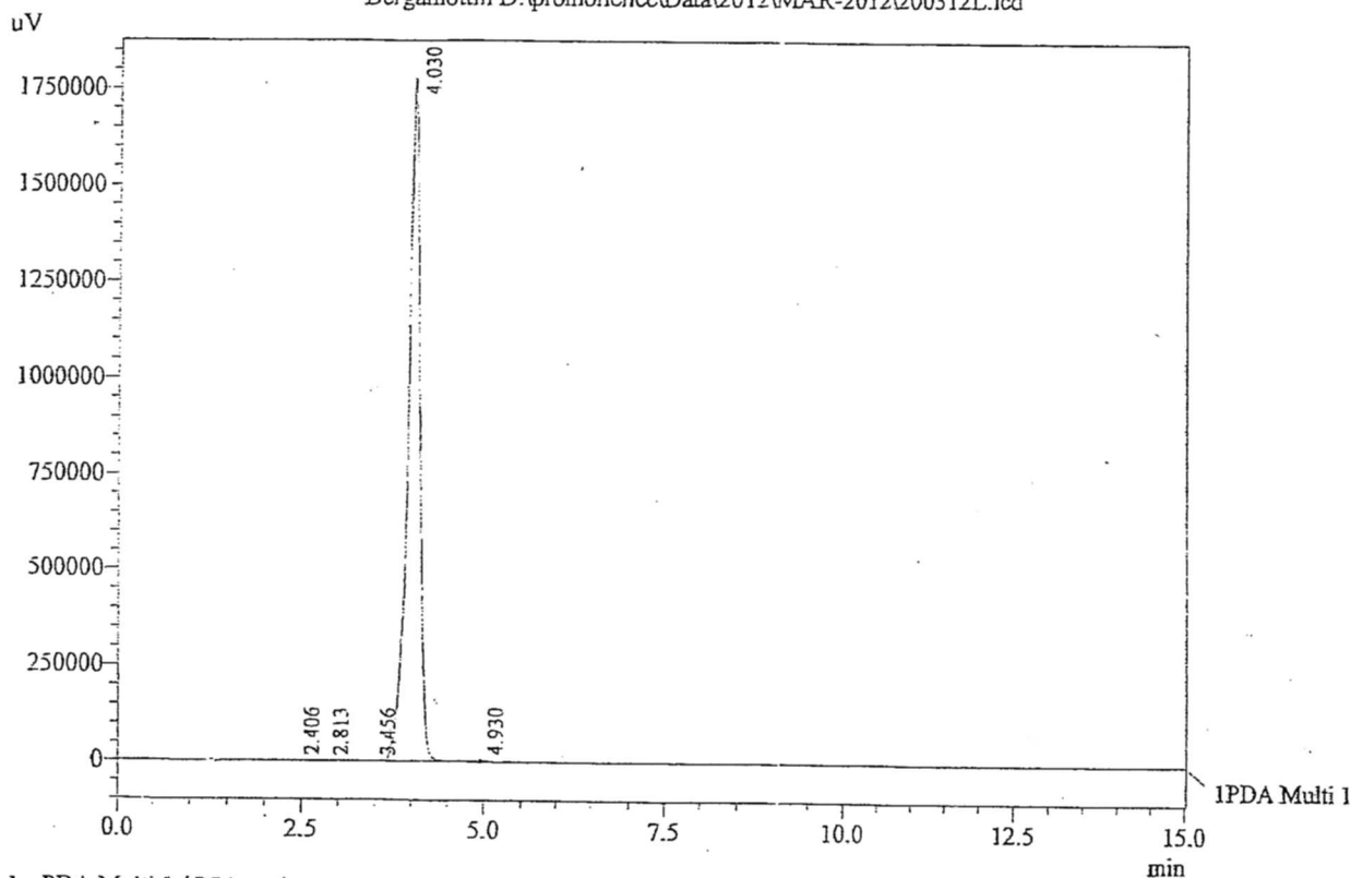
Chromatogram Bergamottin D:\promonence\Data\2012\MAR-2012\200312L.lcd
